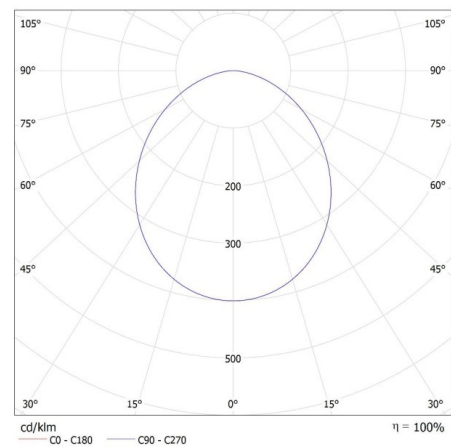
MILEDO (kat 31238) GU10 8W-CW LED / LDC (Polar)
