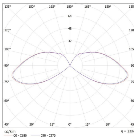
KANLUX S.A. (kat 36556) SELTO 50 B + IQ-LED / LDC (Polar)
