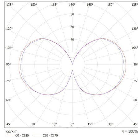
KANLUX S.A. (kat 37241) XLEDIM A60 E27 11W-NW / Krzywa rozsytu światła (biegunowo)
