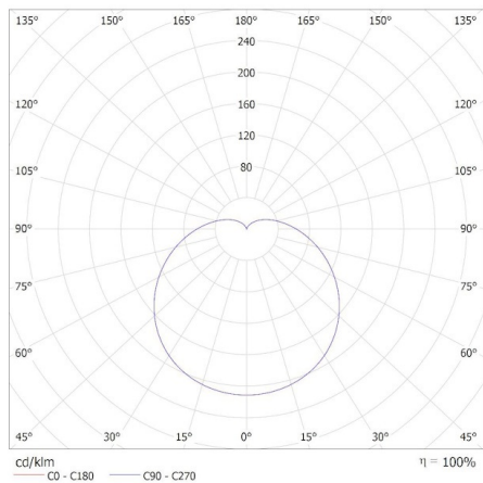
KANLUX S.A. (kat 26768) BILO 6,5W E27-NW / Krzywa rozsytu światła (biegunowo)
