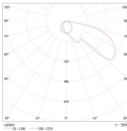
KANLUX S.A. (kat 33691) GLASI LED 3W P WW-B / LDC (Polar)
