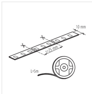
LEDS-B 4.8W/M
