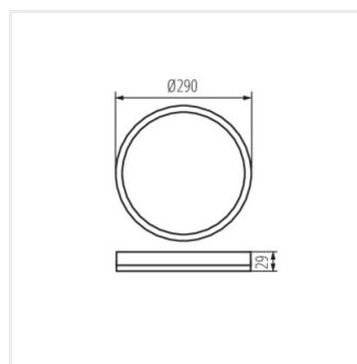
AZPO LED 18,5W-NW-O-B
