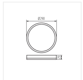
AZPO LED 18,5W-NW-O-B
