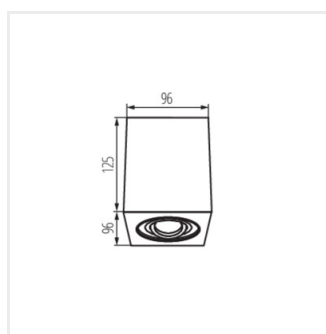
GORD DLP-50
