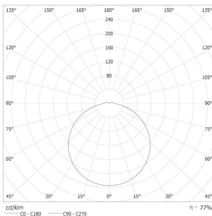
KANLUX S.A. (kat 37297) IPER LED 35W-NW-L / Krzywa rozsytu światła (biegunowo)
