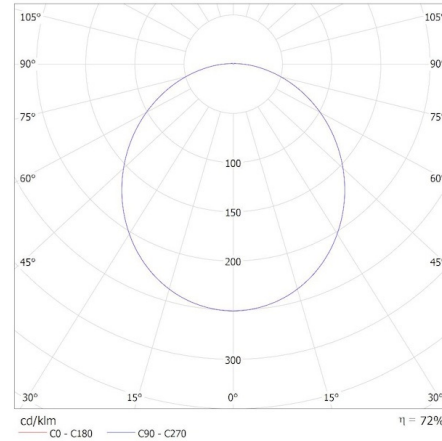
KANLUX S.A. (kat 38777) BENO 12-18W CCT-O-SEW 12W / Krzywa rozsytu światła (biegunowo)
