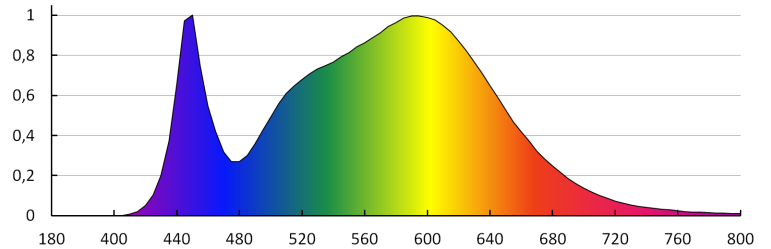
KANLUX S.A. (kat 23423) BILO 6,5W T SMD E14-NW / LDC (Polar)
