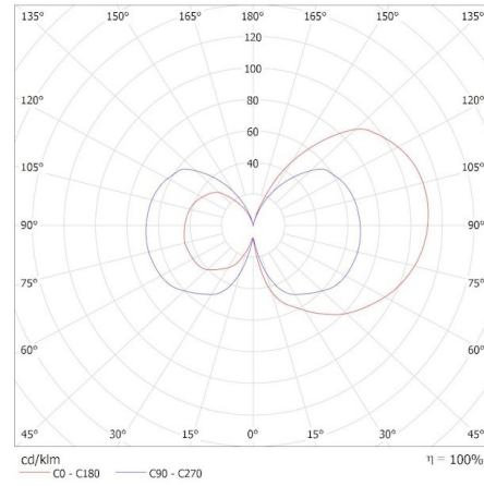
KANLUX S.A. (kat 29606) XLED A60 10W-NW / Krzywa rozsytu światła (biegunowo)
