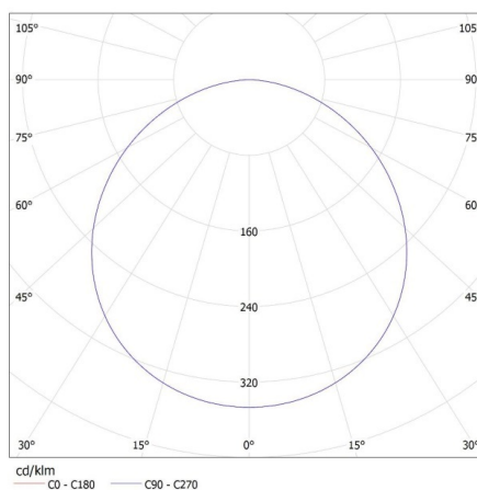
KANLUX S.A. (kat 27210) CARSA V2LED 12W-NW-SN / LDC (Polar)
