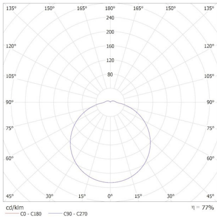
KANLUX S.A. (kat 37301) IPER LED 35W-NW-O-SE / Krzywa rozsytu światła (biegunowo)
