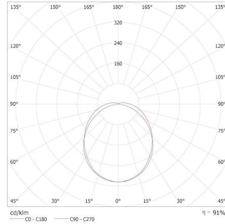
KANLUX S.A. (kat 38463) MAH MAX 19W 06 NW RYF / Krzywa rozsytu światła (biegunowo)
