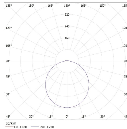
KANLUX S.A. (kat 26441) VARSO LED 18W-NW-O / LDC (Polat)
