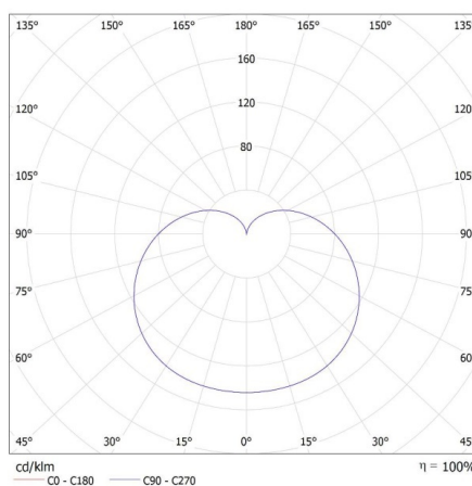
KANLUX S.A. (kat 33734) IQ-LED G45E14 4,2W-WW / LDC (Polar)
