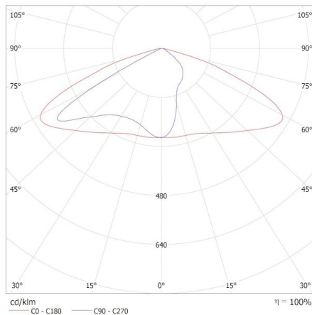
KANLUX S.A. (kat 36228) STRETON LED 20W NW / Krzywa rozsytu światła (biegunowo)
